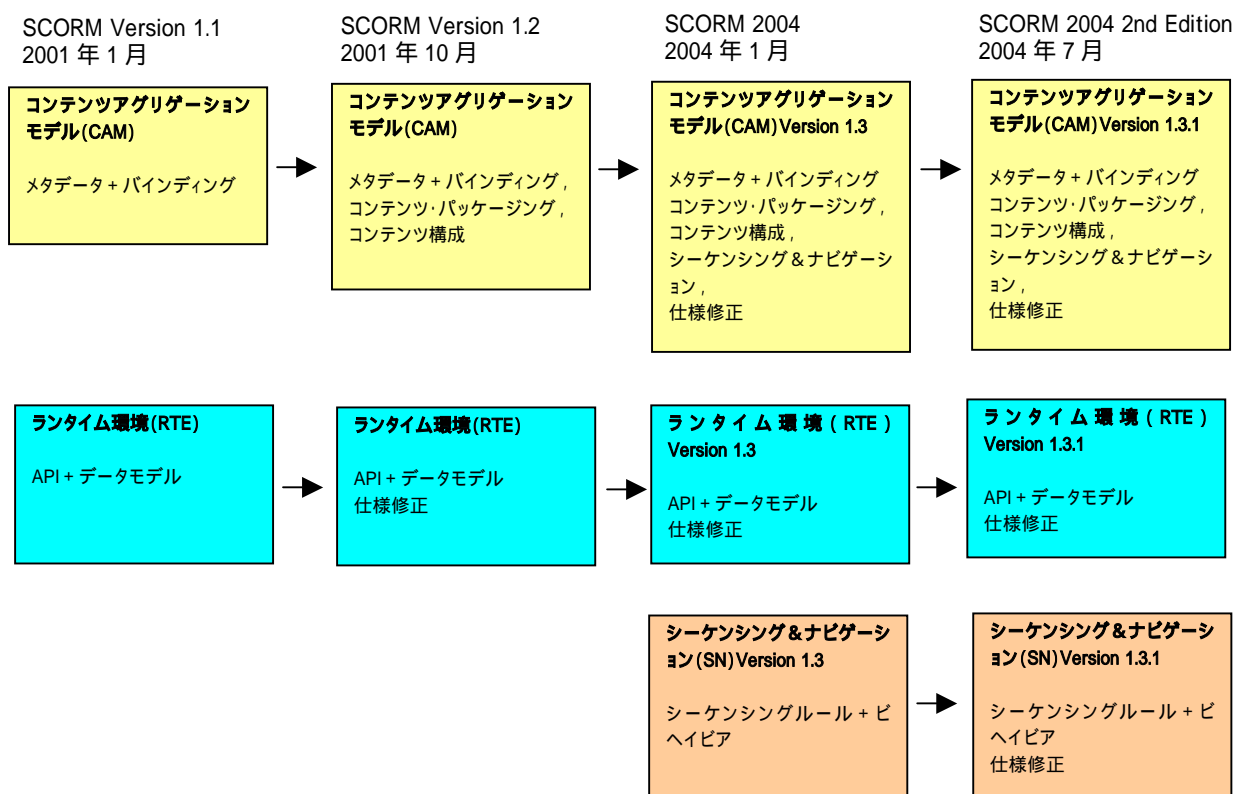
図 2.3 SCORM の進展
